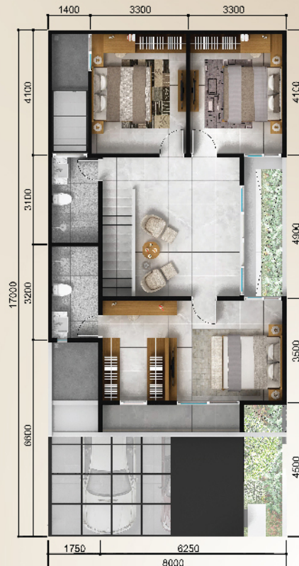
Lantai 2
