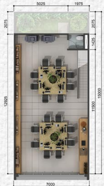
Lantai 3
